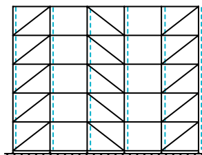
Diagonalstag i vart annat fack, princip A
