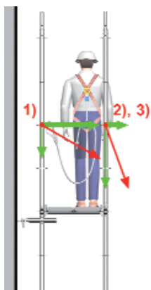
Fig. 3: Anslutningspunkter på kransen (facklängd max. 3,07 m). (OBS! EJ tillåtet på Alu-Allround).
