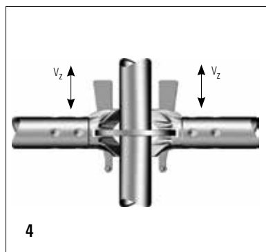
Vertikal skjuvkraft
