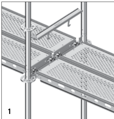
1 och 2. Lägg upp plattformar i U-tvärbommarna och lås dessa mot oavsiktligt lyft.
