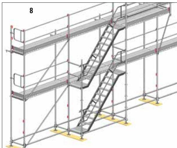
Figur 8. Färdigmonterad STAR
