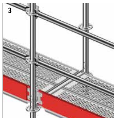
3. Montera ett horisontalstag på 0,5 m höjd över plattformen (mellanliggande ledstång) och på 1,0 m höjd (skydds-räcke). Montera sparklister.
